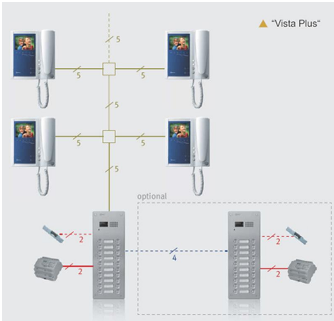
Povezivanje video interfonskog sistema sa 5 žica
