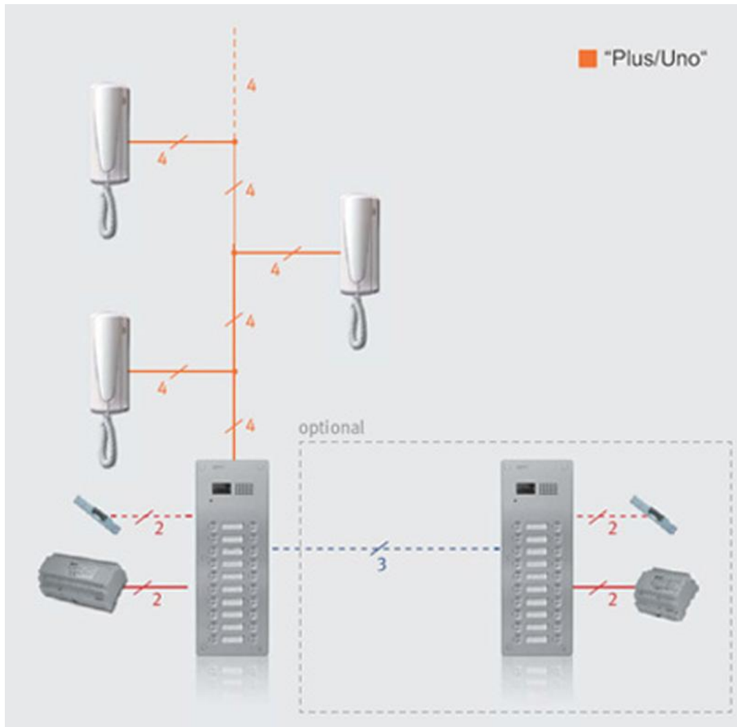
Povezivanje audio interfonskog sistema sa 4 žice
