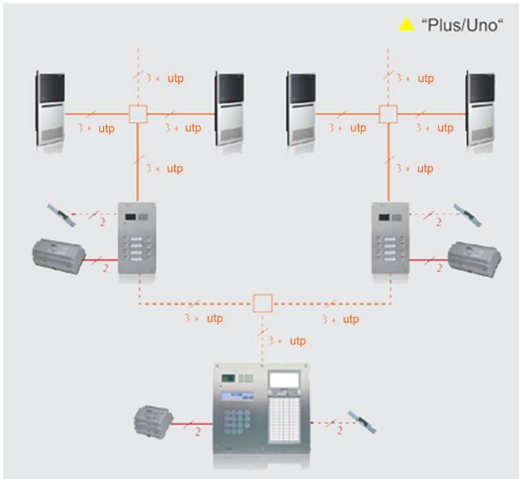
Povezivanje video interfonskog sistema sa 3 žice + UTP
