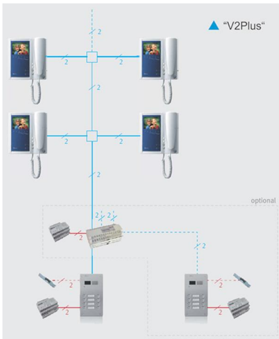
Šema povezivanja video interfona sa 2 žice
