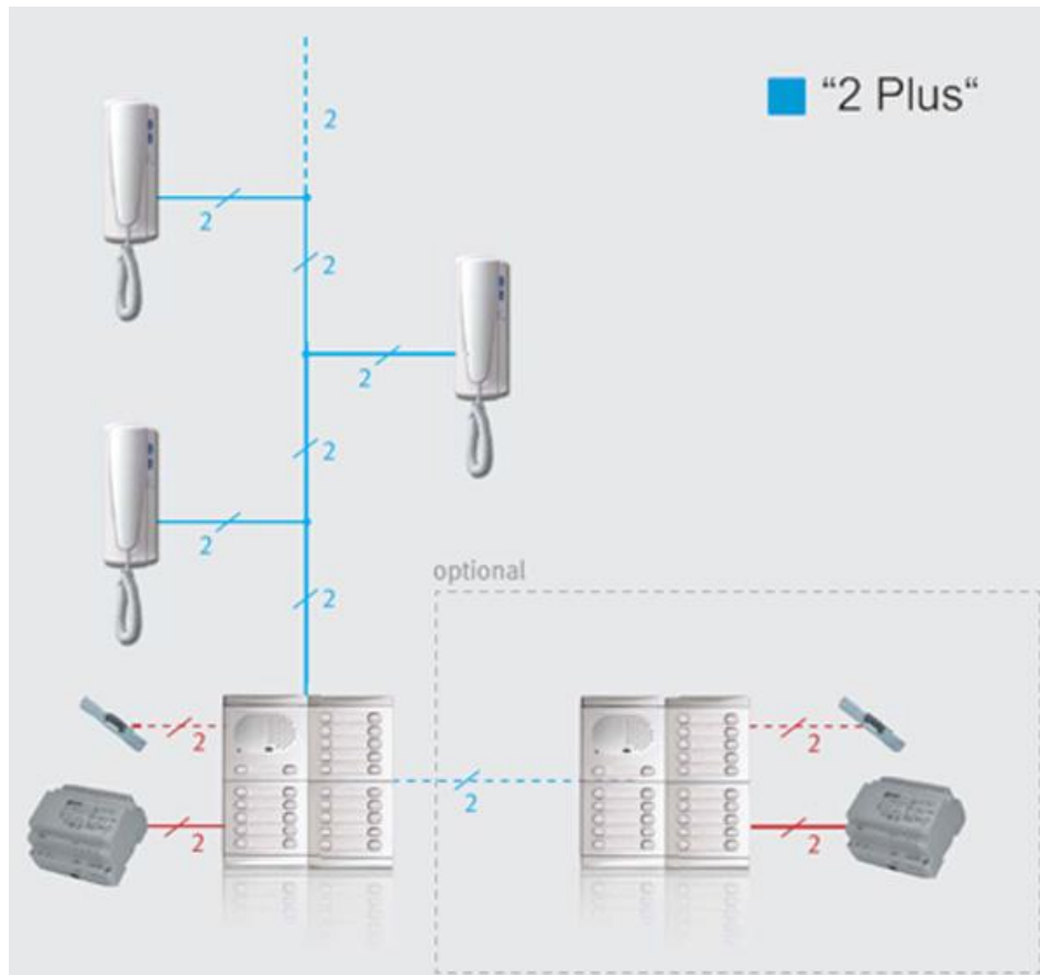
Šema povezivanja audio interfona sa 2 žice
