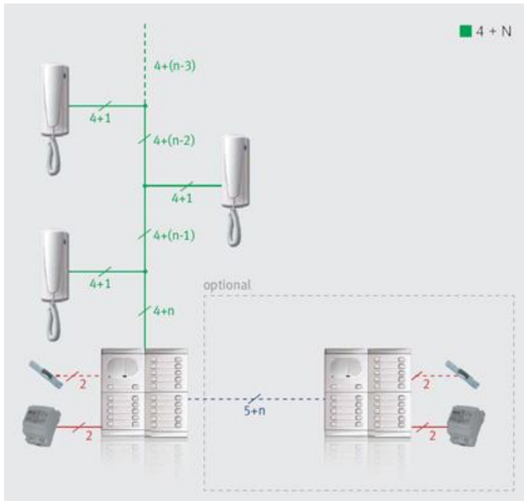
Tradicionalni način povezivanja interfona u zgradama - sa dva ulaza
