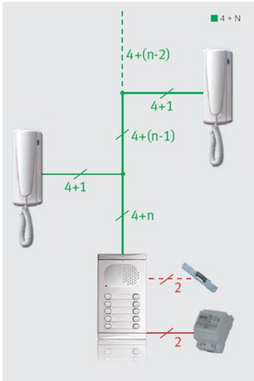
Tradicionalni način povezivanja interfona u zgradama
